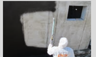
Grundierung eines saugfähigen Untergrunds mit PCI Pecimor® F
