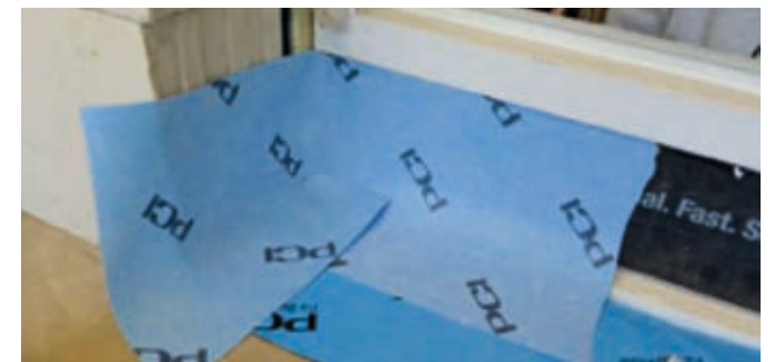
Varianten 2 und 3: mit PCI BT 42 Fixband bzw. PCI Pecitape® 250 in Verbindung mit PCI Barraseal® Turbo abgedichtete Laibungsflächen sind leicht überputzbar und haftungsfreundlich
